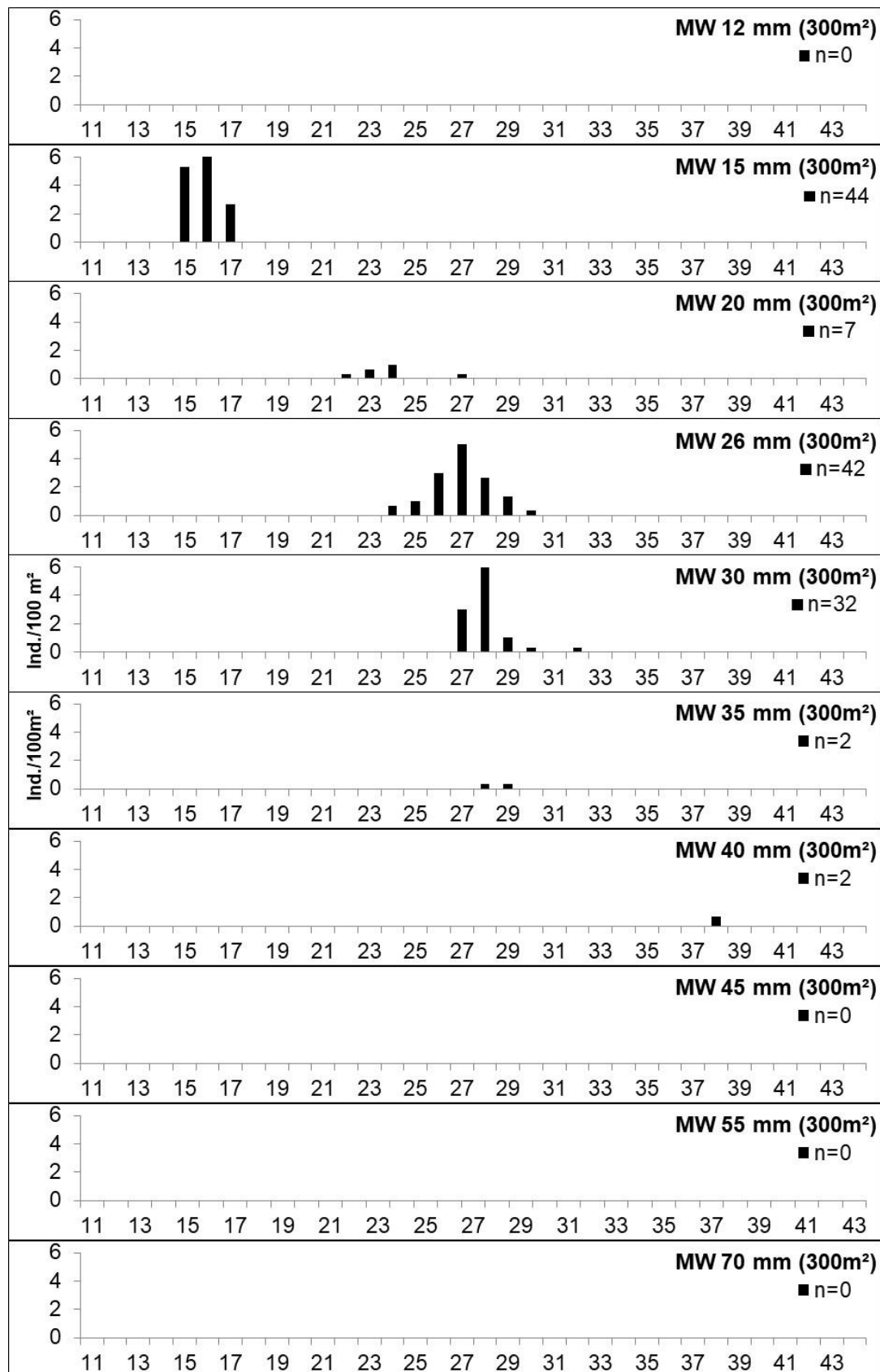
Abb. 5: Längenhäufigkeitsverteilung der im November 2022 gefangenen Reinanken pro verwendeter Kiemennetzmaschenweite und 100 m² Netzfläche. In Klammer ist die gesetzte Netzfläche pro Maschenweite angegeben.
