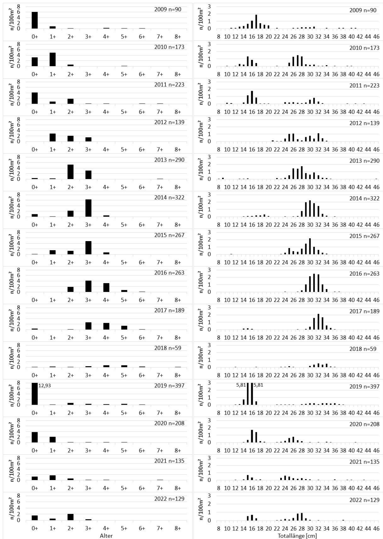
Abb. 11: Alterklassenverteilung und Längenfrequenzen von Renken in den Jahren 2009 bis 2022 bezogen auf eine einheitliche Netzfläche von 100 m 2 .
