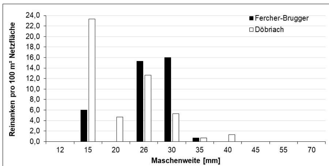
Abb. 4: Gefangene Reinanken pro Maschenweite und Befischungsbereich bezogen auf 100 m² Netzfläche
