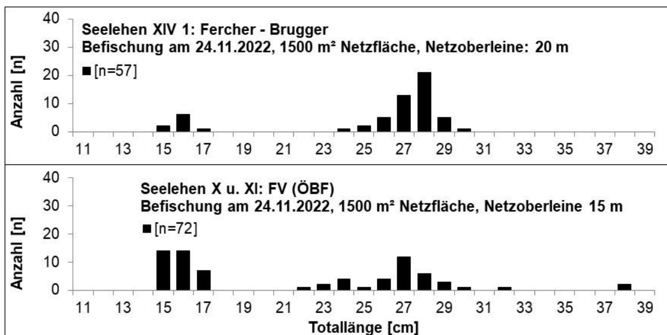
Abb. 3: Längenhäufigkeitsverteilung von Reinanken die im Lehen Fercher-Brugger (Bereich Lagerbucht; oben) und im Lehen Fischereiverband Millstätter See (Bereich Döbriach; unten) am 24.11.2022 gefangen wurden.
